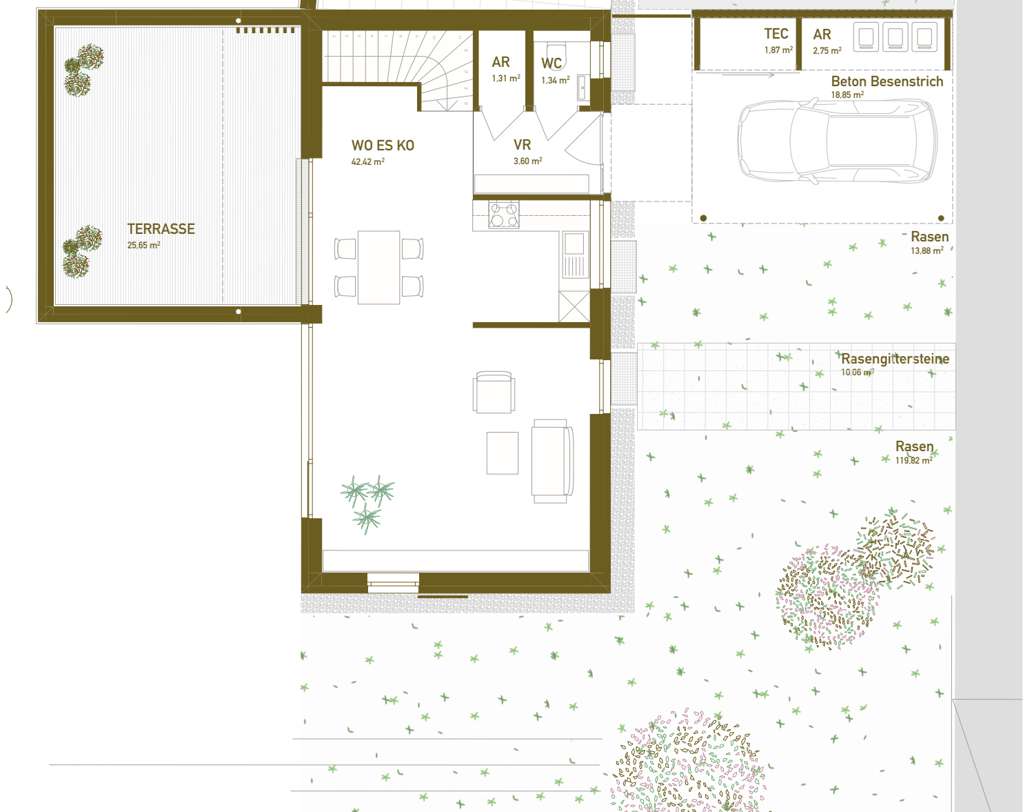
GRUNDRISS EBENE 00 M 1:100
