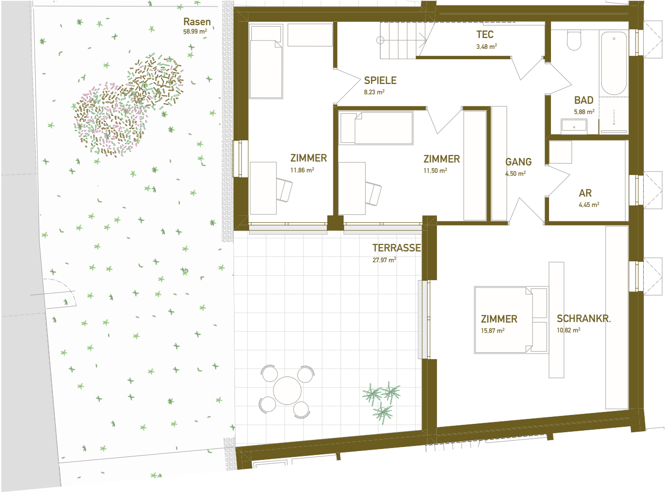
GRUNDRISS EBENE -01 M 1:100
