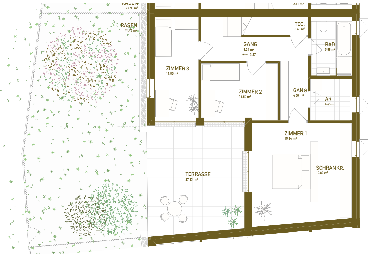
GRUNDRISS EBENE -01 M 1:100
